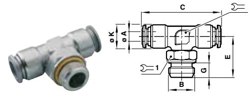
T-Verschraubung, drehbar
