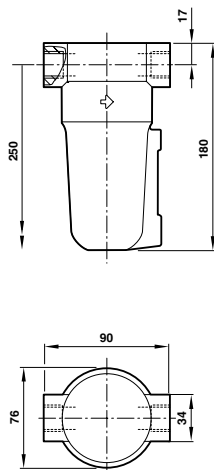
F22 Manuelle Entleerung
