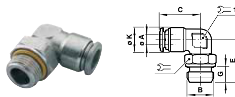
Winkelverschraubung, drehbar
