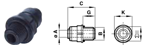
Gerade Einschraubverschraubung
