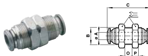
Gerade Schottverbindung
