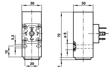
Flansch
