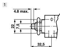
Tastrolle, vorgesteuert – G1/8-Ventile
