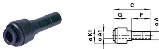
Gerade Reduzier-Steckverbindung (Stutzen/Schlauch)
