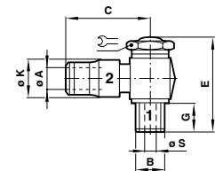
Drosselrückschlagventil (Abluft), Einstellschraube versenkt
