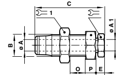
Kombinierte Schottverbindung (Push-In auf Klemmring)
