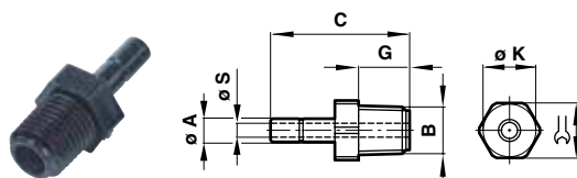
Einschraub-Steckstutzen
