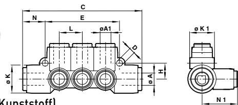
Mehrfachverteiler (Kunststoff)
