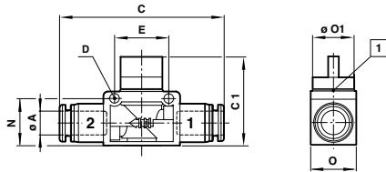
Absperrventile (Anschluss: Rohr/Rohr)
