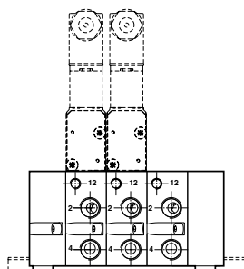
Anschlüsse 2+4 seitlich
