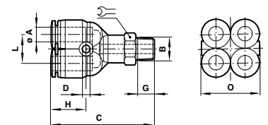
Mehrfachverteiler, 4-fach
