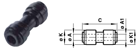
Gerade Reduzierverbindung
