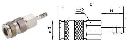
Kupplungsdose mit Schlauchanschluss
