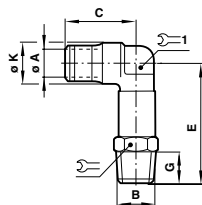
Winkelverschraubung drehbar, lang
