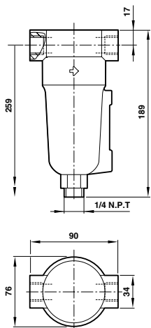
F22 Automatische Entleerung
