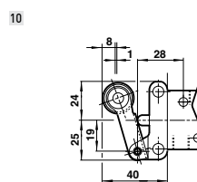
Tastrolle, verstärkte Ausführung – G1/8-Ventile
