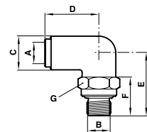
Universal-Winkelverschraubung
