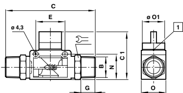
Absperrventile (Anschluss: Gewinde/Gewinde)
