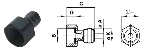
Gerade Aufschraubverschraubung
