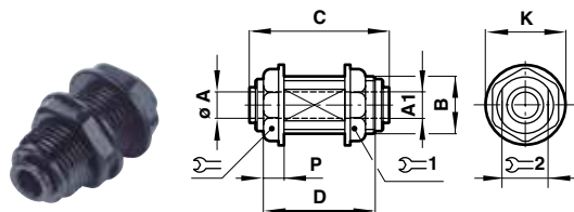
Gerade Schottverbindung
