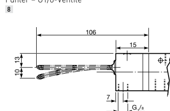
Fühler – G1/8-Ventile
