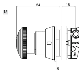
Notknopf – G1/8-Ventile
