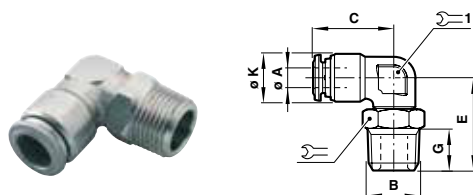
Winkelverschraubung, drehbar
