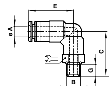
Winkelverschraubung, absperrend
