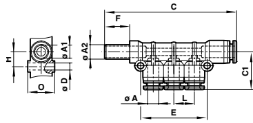
Mehrfach-Steckverteiler
