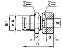
Gerade Aufschraub-Schottverschraubung (Innengewinde)
