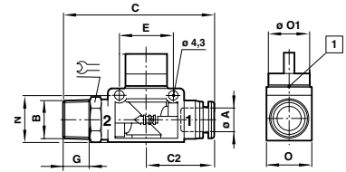
Absperrventile (Anschluss: Rohr/Gewinde)
