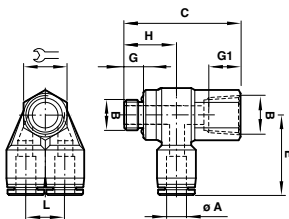
Mehrfach-Einschraubverteiler
