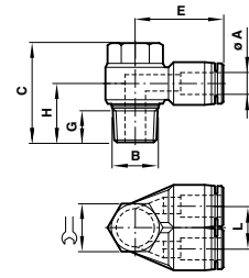
Schwenkverschraubung, 2-fach
