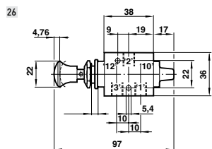
Knopf mit Knopf-Rückstellung - G1/8-Ventile
