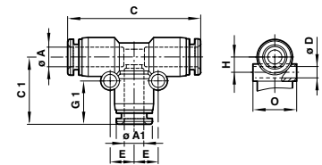
T-Reduzierverbindung
