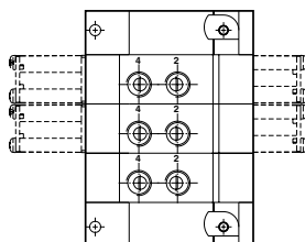
Anschlüsse 2+4 unten
