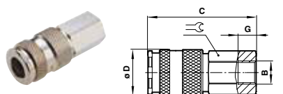
Kupplungsdose mit Innengewinde
