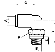
Winkelverschraubung drehbar
