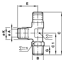
Y-Verschraubung (Kunststoff)
