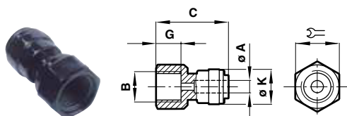
Gerade Aufschraubverschraubung
