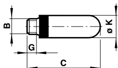
Einschraub-Ausführung
