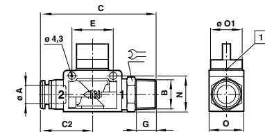
Absperrventile (Anschluss: Gewinde/Rohr)
