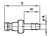
Kupplungsstecker mit Schlauchtülle
