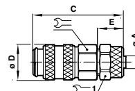
Kupplungsstecker mit Push-on-Verschraubung
