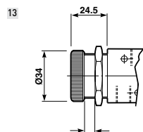
Knopf (Schutzkragen) – G1/8-Ventile
