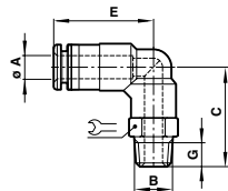
Winkelverschraubung, absperrend
