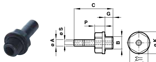
Einschraub-Steckstutzen
